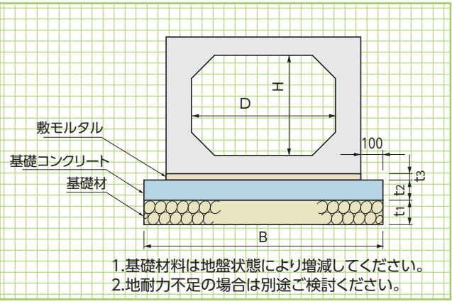
■コンクリート基礎工による標準敷設材料表 (10m当り)
