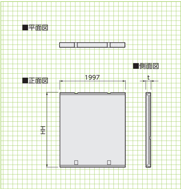
基本形状図
