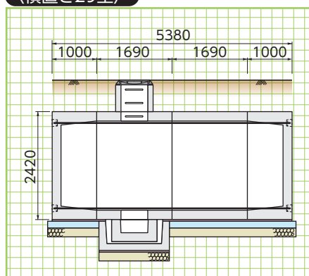
〈横置き29型〉
