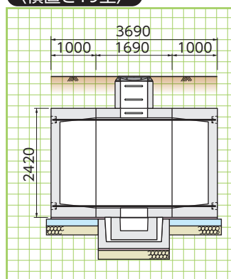
〈横置き19型〉
