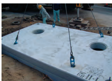
頂版敷設
