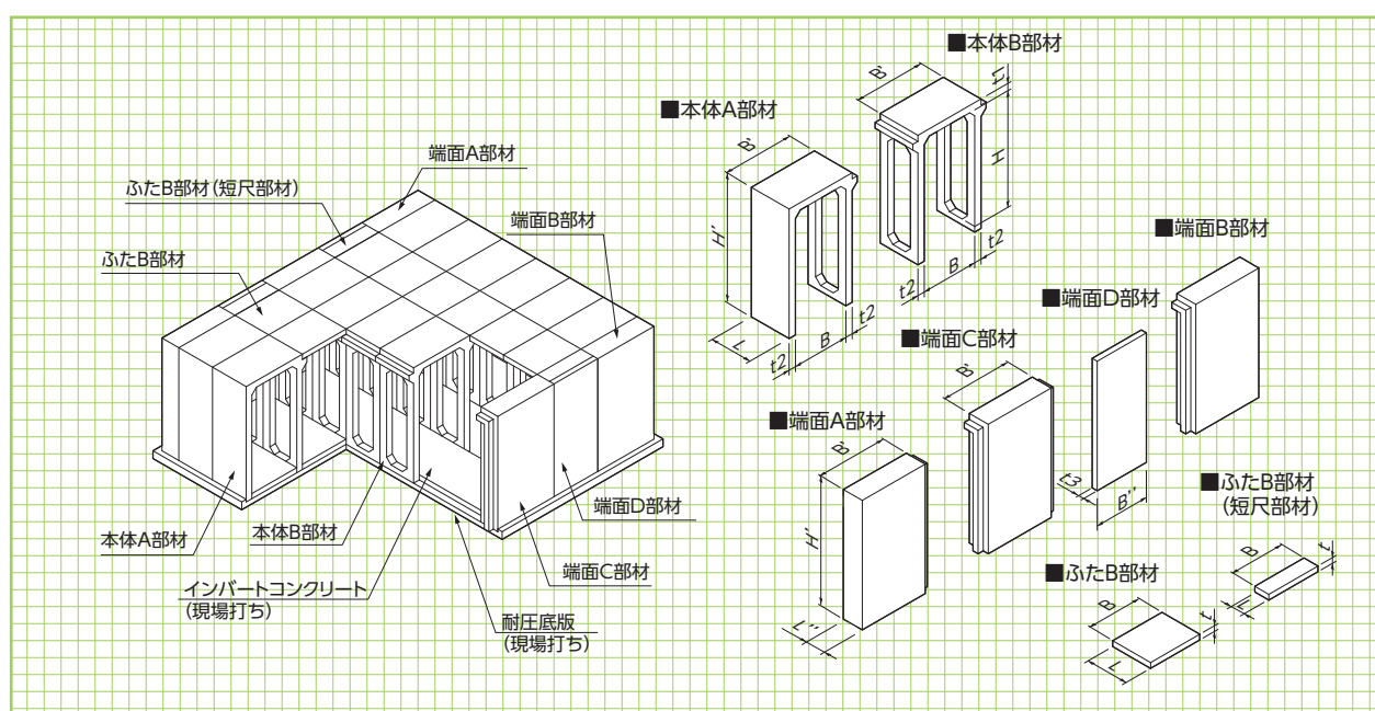
■寸法・重量表(本体部材、端面部材)
