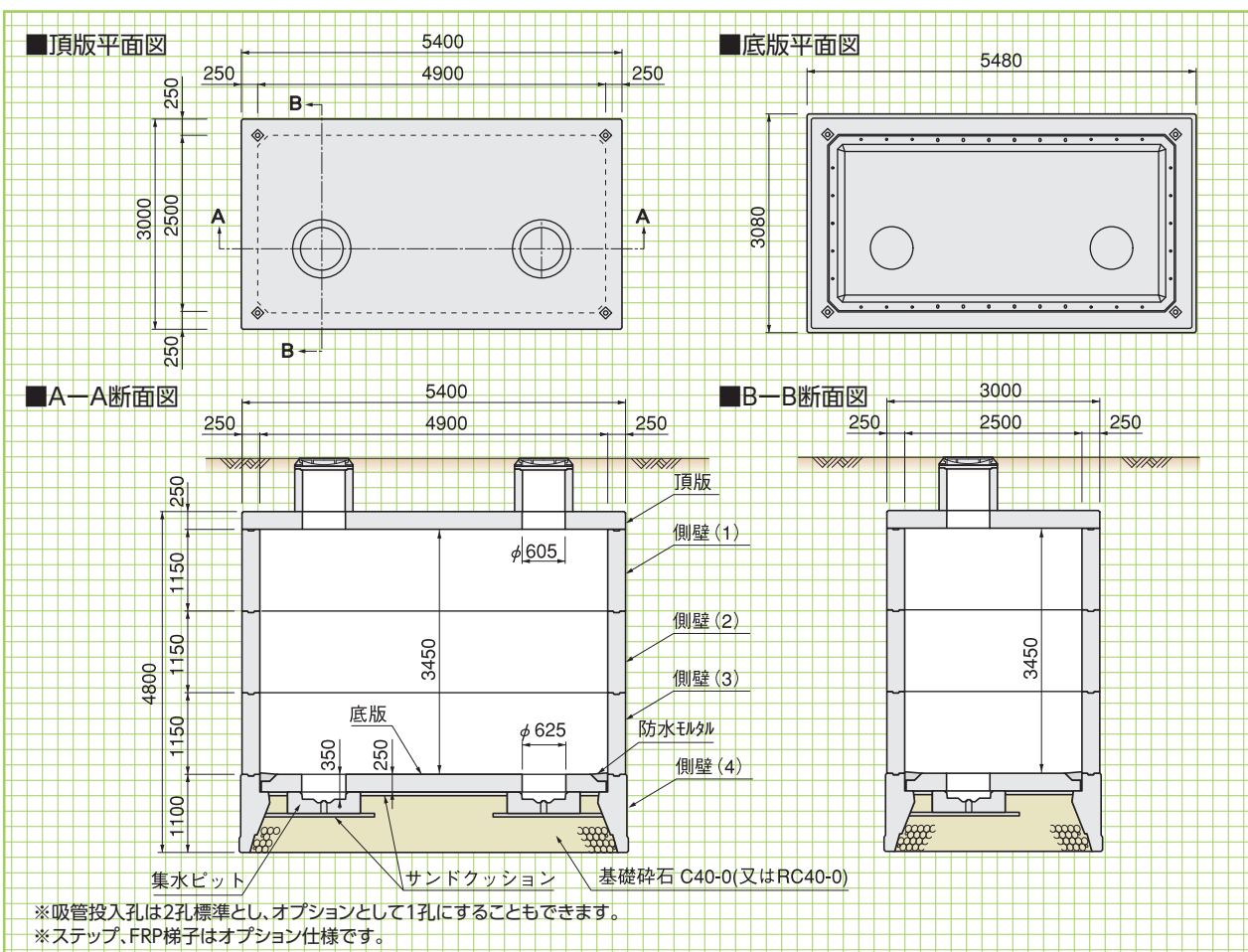
基本形状図
