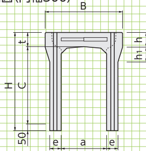
■正面図(内幅300)
