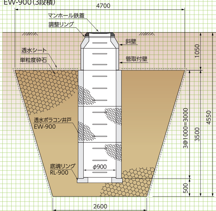
■標準施工断面図 EW-900(3段積)
