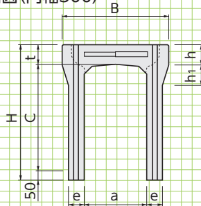
■正面図(内幅300)
