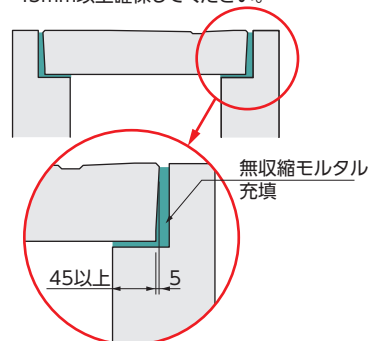
基本形状図 形状・寸法
