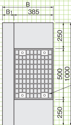
■平面図
