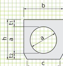
■A-A' 断面図
