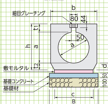
■A-A' 断面図
