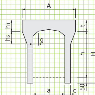
■B-B'断面
