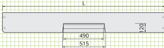
■側面図
