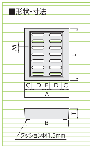
基本形状図
