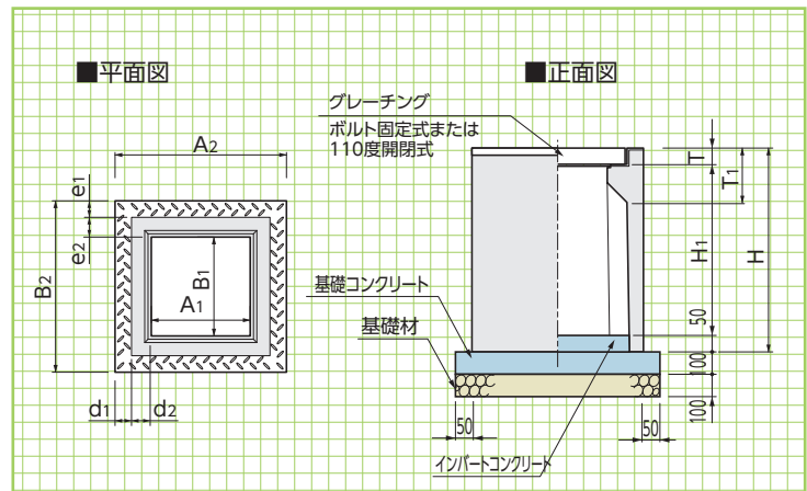
■寸法・重量表(AS型柵) ※印は特注扱いになりますので、営業担当にお問い合わせください。
