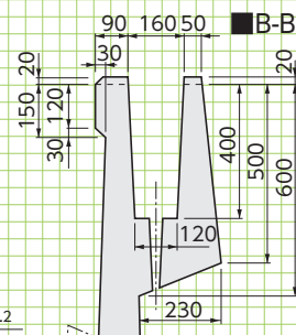
■B-B'断面図
