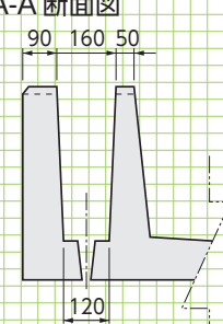
■A-A'断面図
