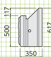
■側面図
