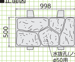
■正面図
