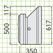
■側面図
