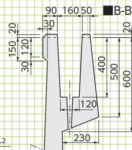
■B-B'断面図
