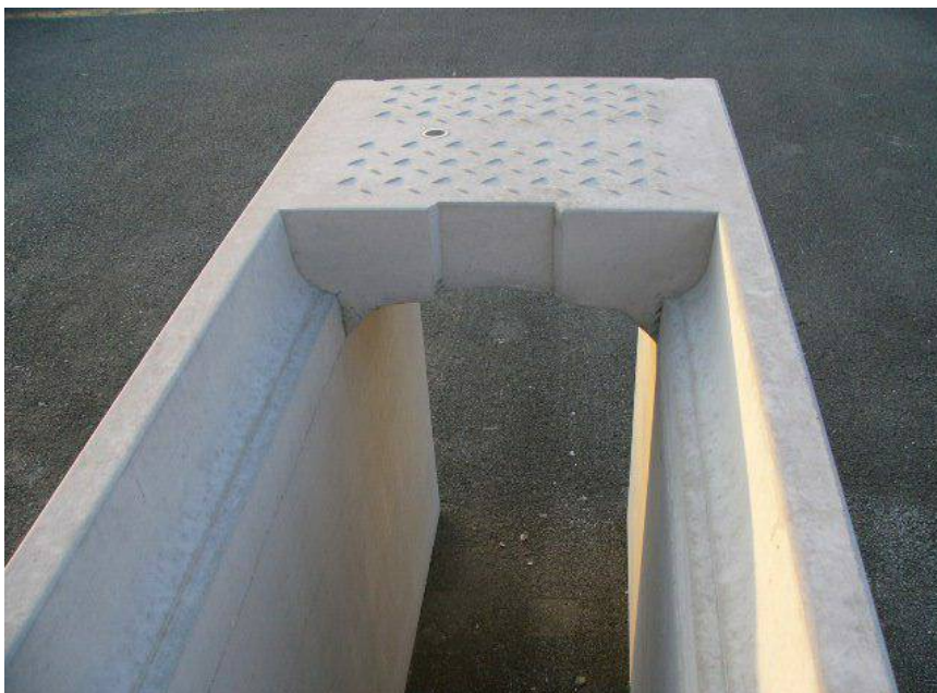
リボーン側溝単体04
