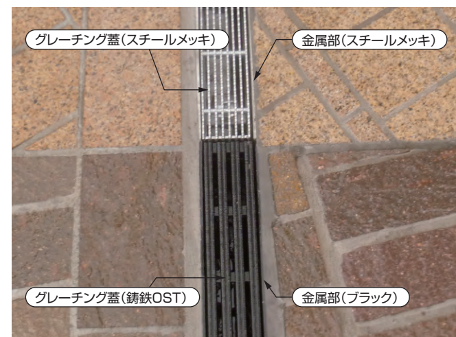
▲金属部分とグレーチング
