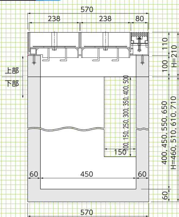
柵断面図 直線用
