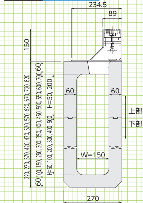
溝断面図 L=2000,L=1000
