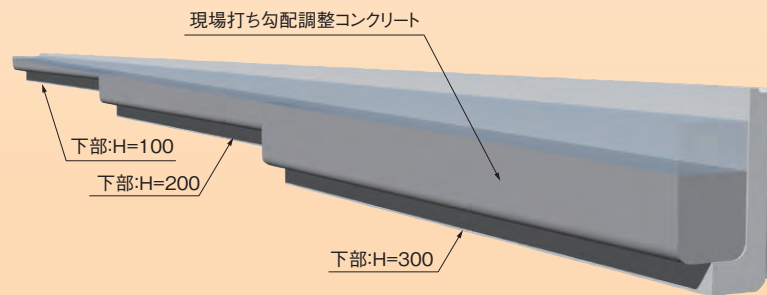
可変側溝使用例イメージ
